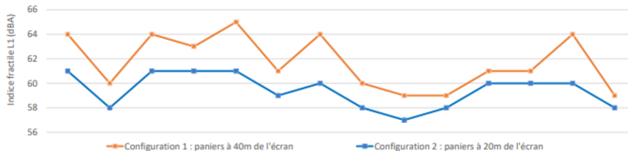
Niveaux sonores à Anglet lors des lâchers de ferraille dans les paniers suivant 2 configurations
