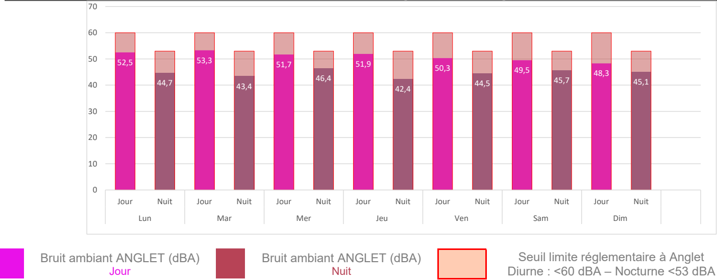
Niveaux sonores enregistrés à Anglet (dBA)
